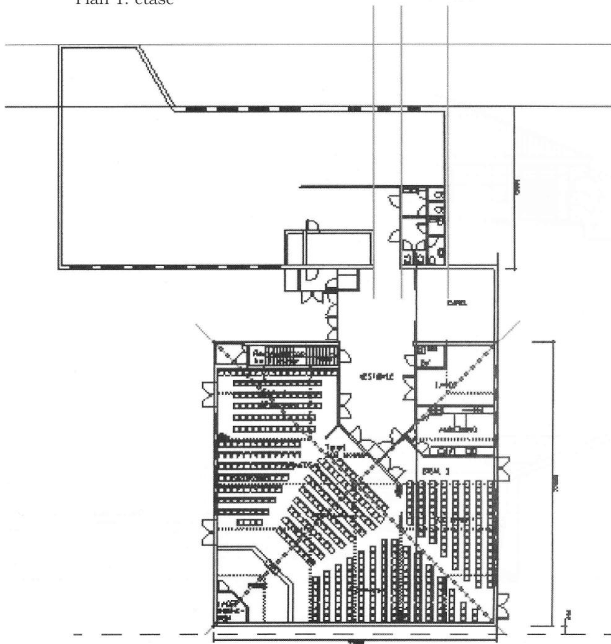
Plan 1. etase
